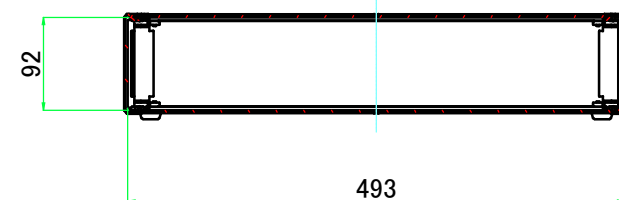
B-B ( 1 : 7.5 )
